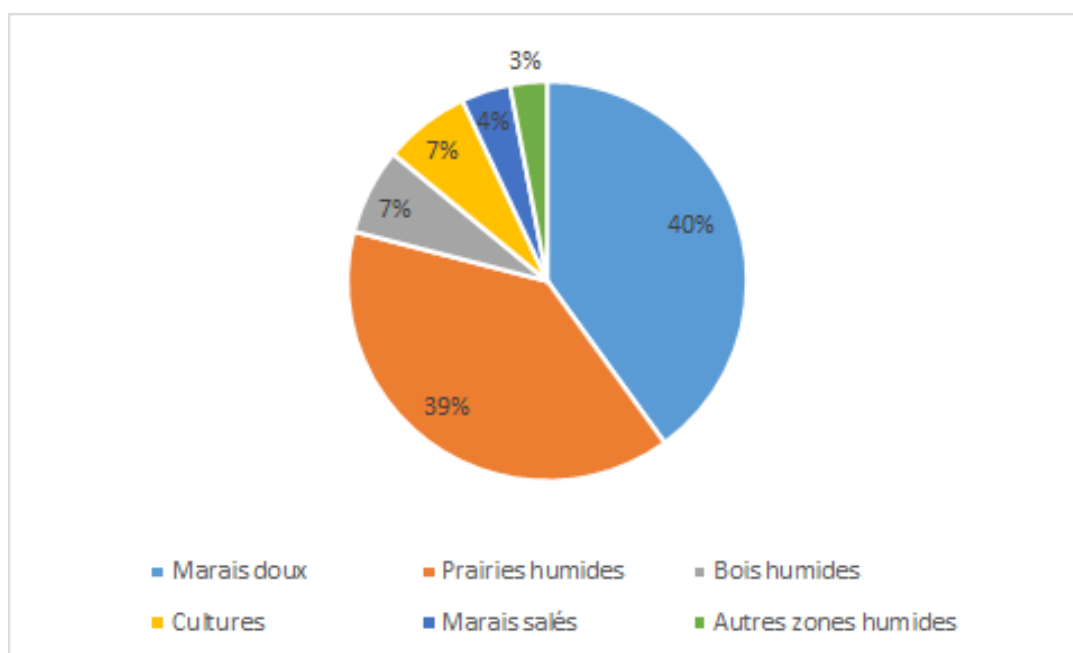
Figure 33: les types de zones humides sur le bassin versant de la Vie et du Jaunay (source : inventaire SAGE)
